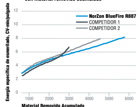
Energía específica de esmerilado comparado con material removido acumulado
