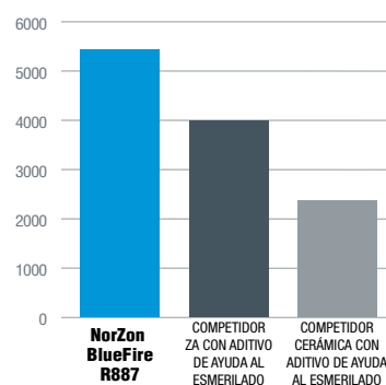
304 SS remoción de material
