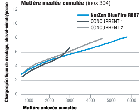
Charge spécifique de meulage c. Matière meulée cumulée (inox 304)
