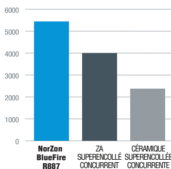
Enlèvement de matière - inox 304
